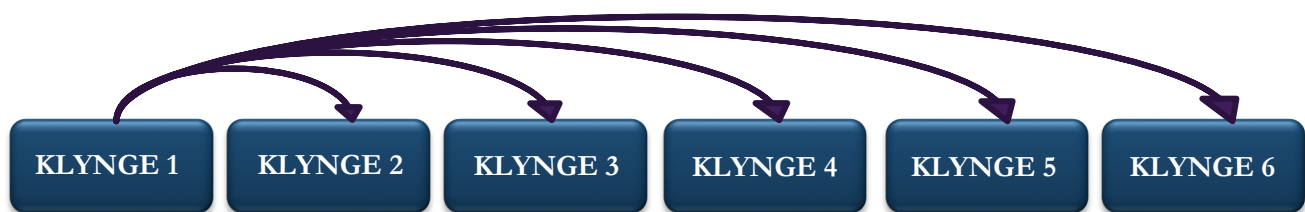
Figur 3: Eksemplificering af fremgangsmåden ved brug af multinomial logistisk regression
