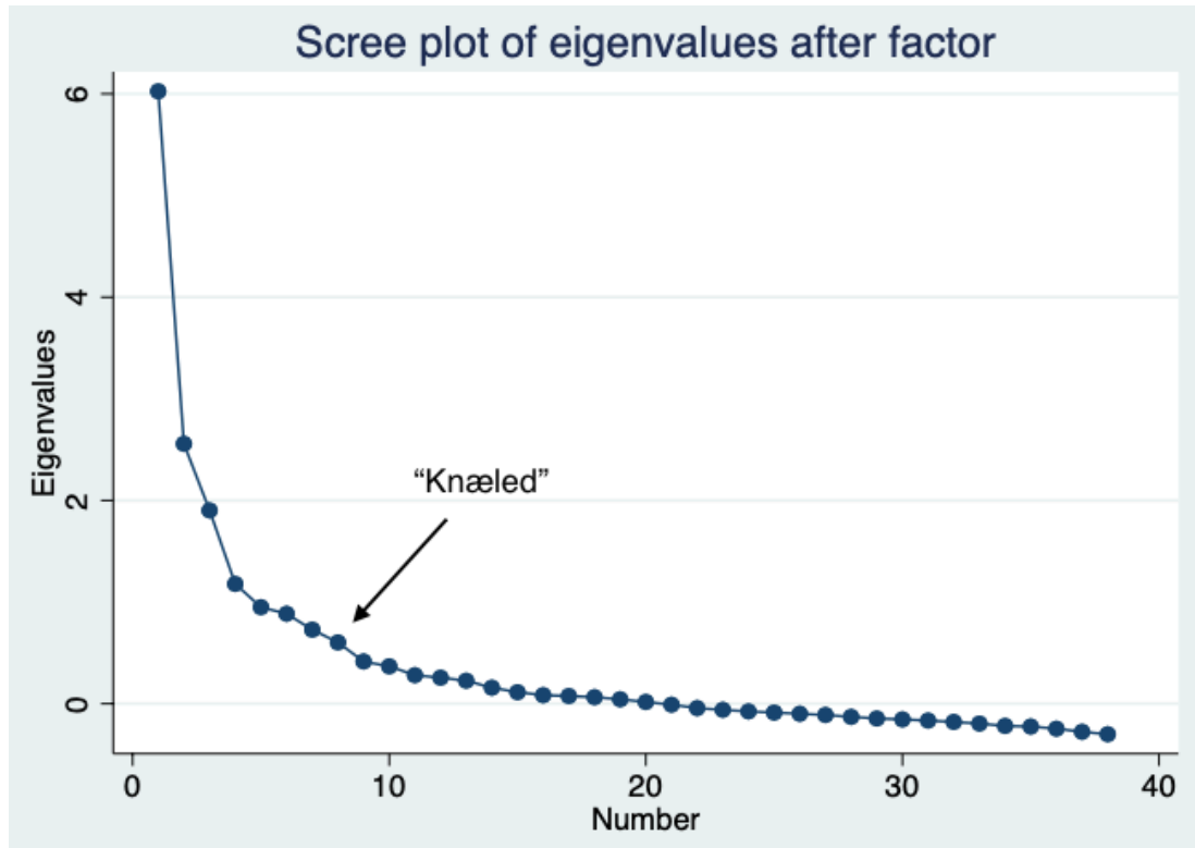
Figur 3: Screeplot af egenværdierne før rotation
