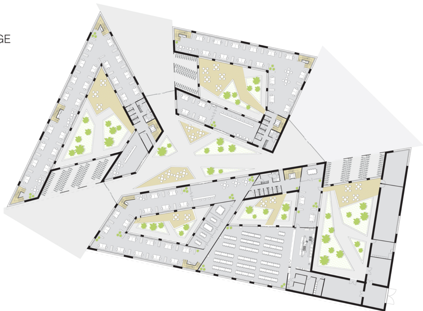
FØRSTEETAGE 1:750
