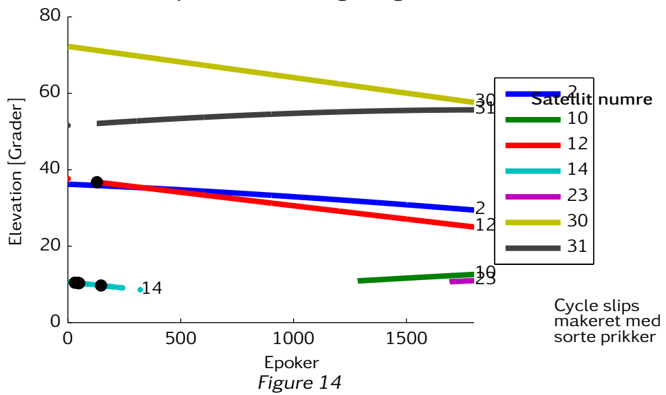
Elevationsplot "mm" forsøg, Magellan AC12
