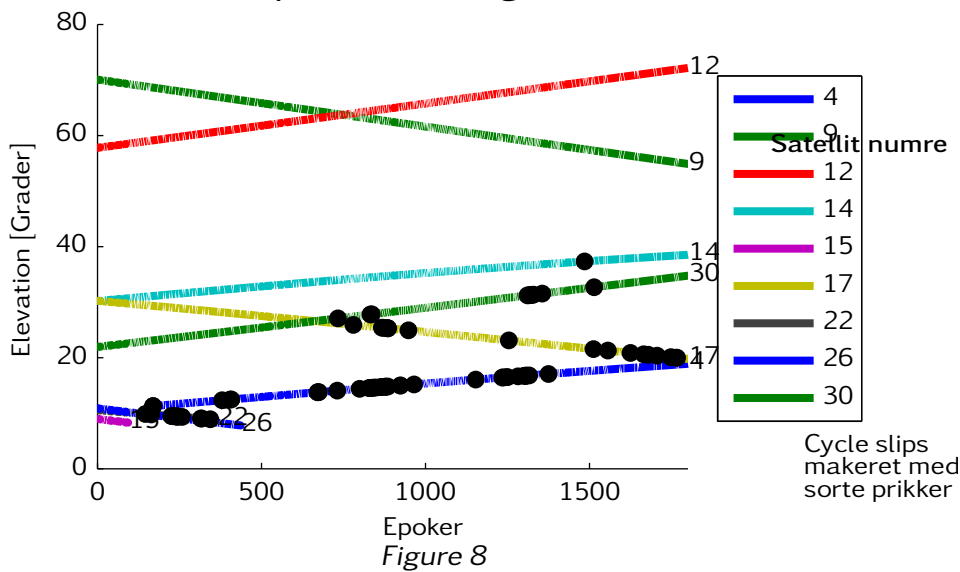
Elevationsplot "mu" forsøg, Garmin 12XL
