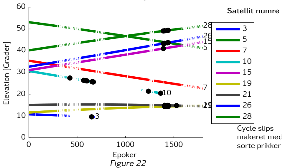
Elevationsplot "1k" forsøg, Antaris LEA 4T
