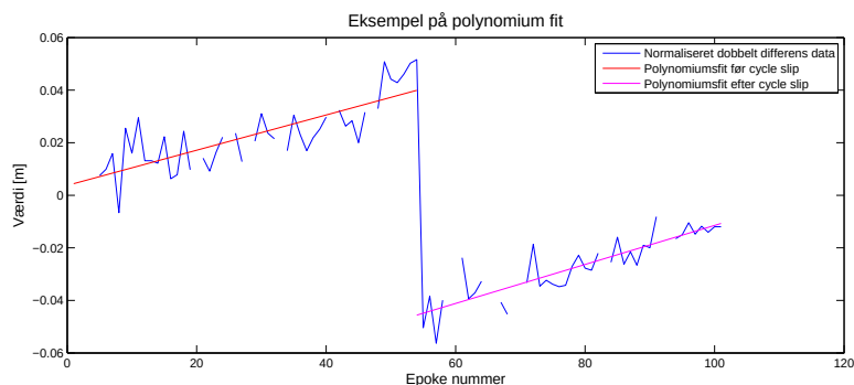
Figur 2.2: Viser eksempel på polynomiumsfit.
