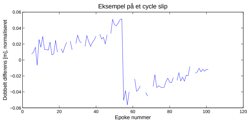
Figur 2.1: Viser et hop i dobbelt differentieret data - et cycle slip.
