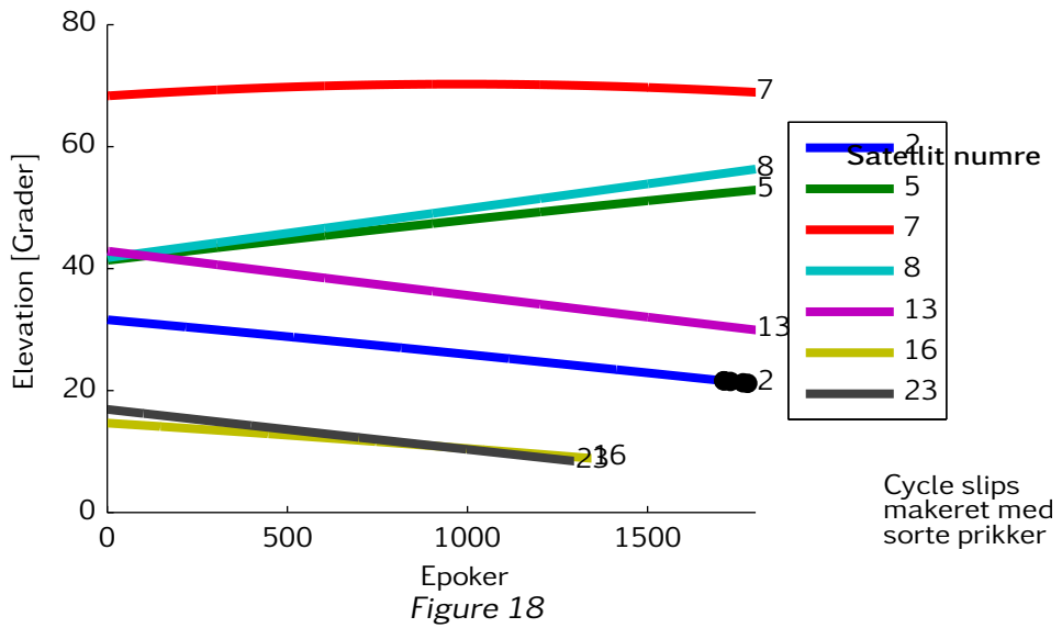
Elevationsplot "d5" forsøg, Antaris TIM-LP
