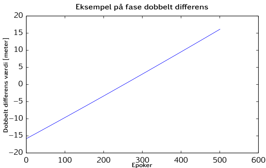
Figur 4.1: Viser et eksempel på dobbelt differentieret data for en enkelt satellit. Data er normaliseret ved at fratrække middelværdien for de 500 epoker.
