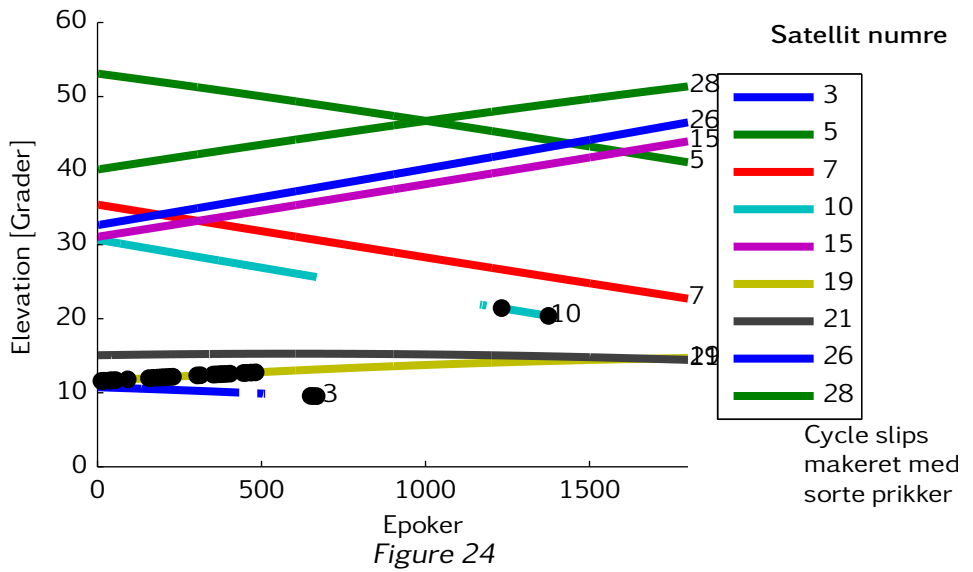
Elevationsplot "1k" forsøg, Antaris TIM-LP
