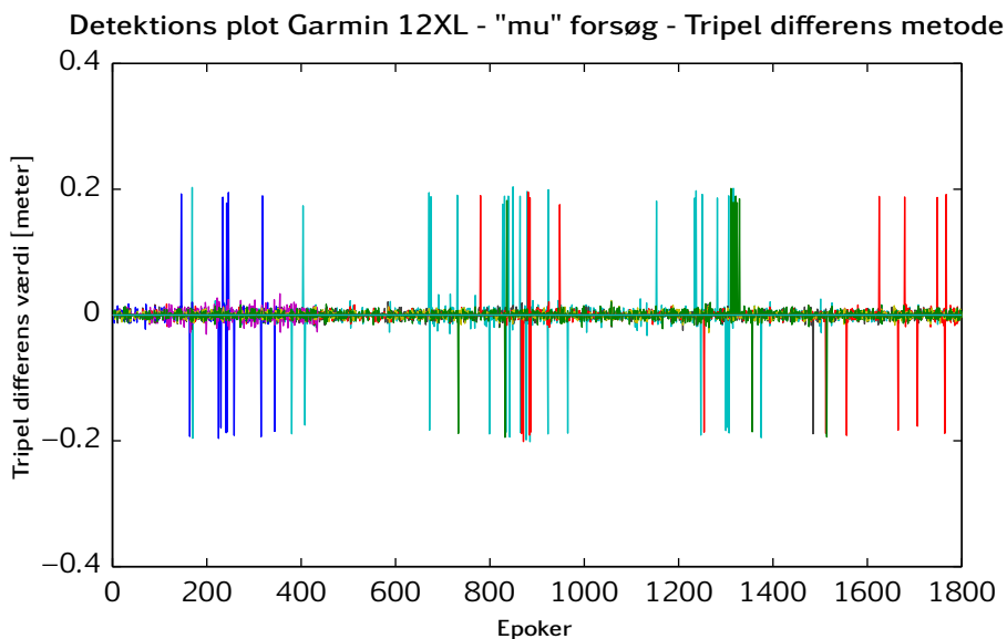
Figur 6.14: Viser de 79 cycle slips der detekteres i forsøget.
