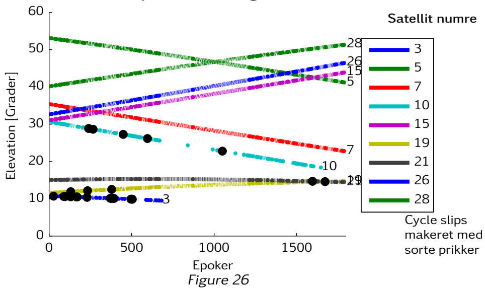
Elevationsplot "1k" forsøg, Garmin 12XL
