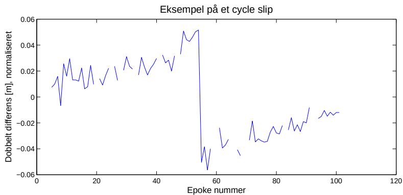
Figur 4.2: Viser et hop i dobbelt differentieret data. Bemærk de huller der er i datasættet omkring cycle slippet.
