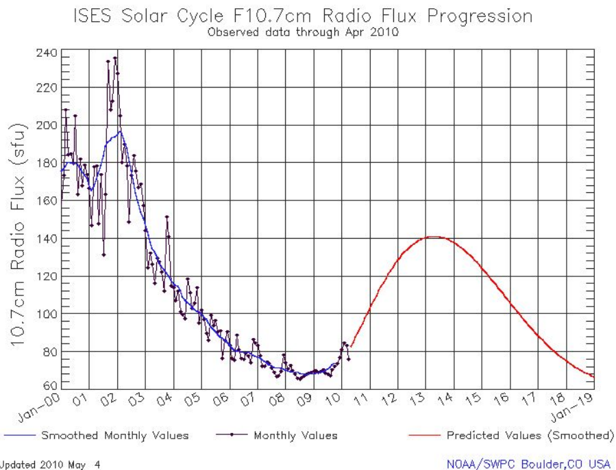
Figur 4.4: Viser de solspot aktiviteten fra år 2000 til 2010 [5].
